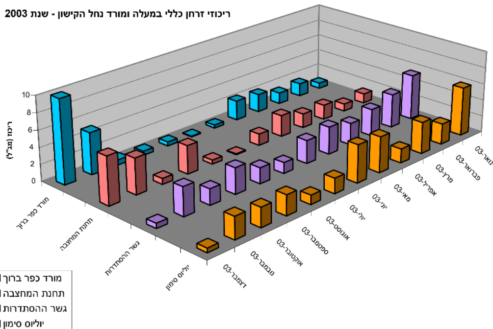
זרחן כללי ברציף האבן וביובלי הקישון - שנת 2003
