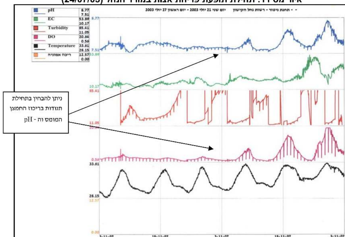
איור מס' 11: תחילת תופעת פריחת אצות במורד הנחל (24/07/03)
