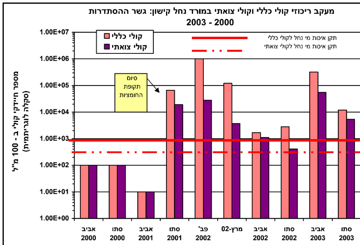
איור מס' 7: מעקב ריכוזי קולי כללי וצואתי בתחנת הדיגום "גשר ההסתדרות" בשנים 2000 - 2003
