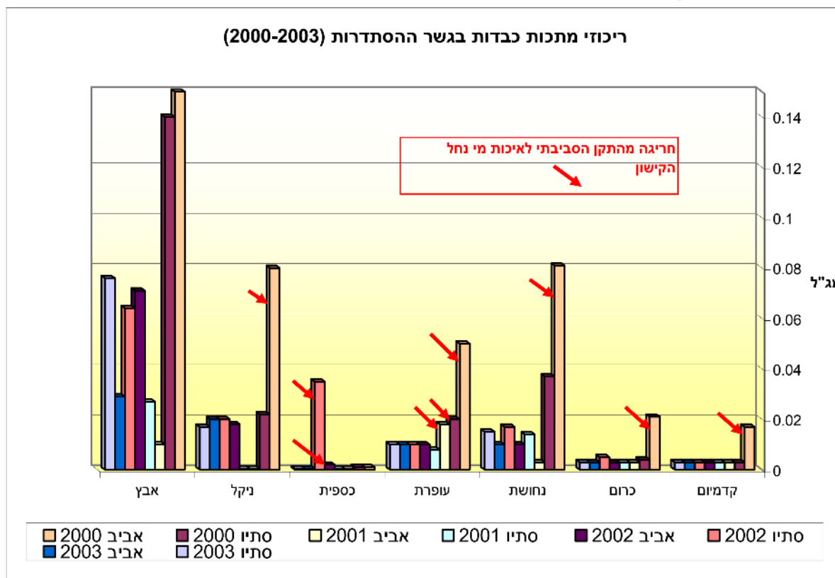
איור מס' 8: מעקב ריכוזי מתכות כבדות בתחנת דיגום "גשר ההסתדרות" בשנים 2000 - 2003
